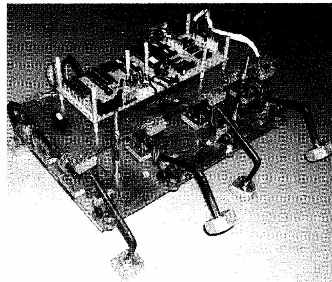
אחד מהרובוטים בפרויקט האלקטרוניקה. בזכות המורה התלמידים יישאו עמם מורשת לחיפוש פתרונות יצירתיים
